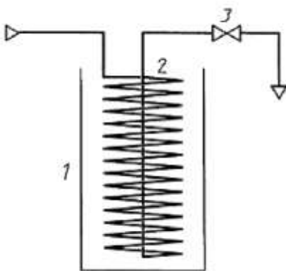
1 — сосуд для охлаждающей смеси; 2 — змеевик; 3 — игольчатый вентиль
