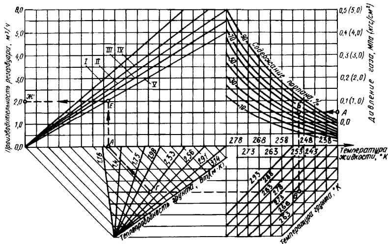
Номограмма для определения производительности резервуара сжиженного газа вместимостью 2,5 и 5 м³ (подземного)
